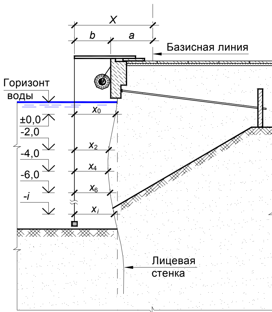
Рисунок 8.1 – Схема измерений наклона (прогиба) лицевой стенки сооружения Т а б л и ц а 8.1 – Положение лицевой стенки сооружения
